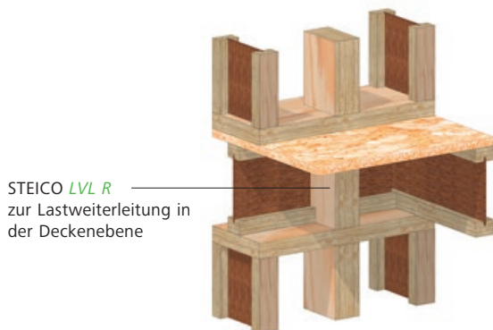
F5 Weiterleitung hoher Einzellasten durch die Deckenebene
