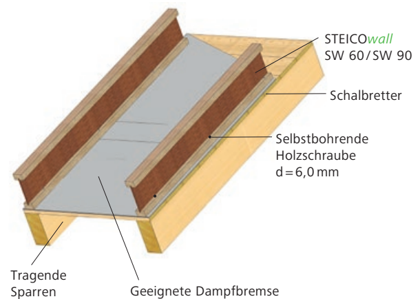
D12 Aufdachdämmung – Aufdoppelung mit STEICOwall
