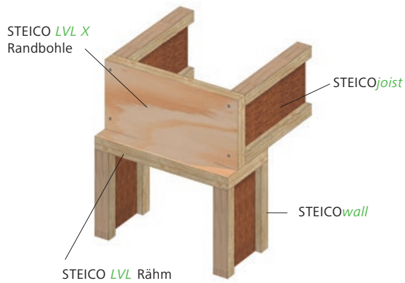
F1 Deckenanschluss mit Randbohle
