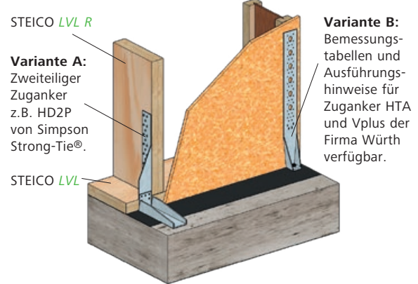
Abdichtung und Detailausbildung nach DIN 68800-2
